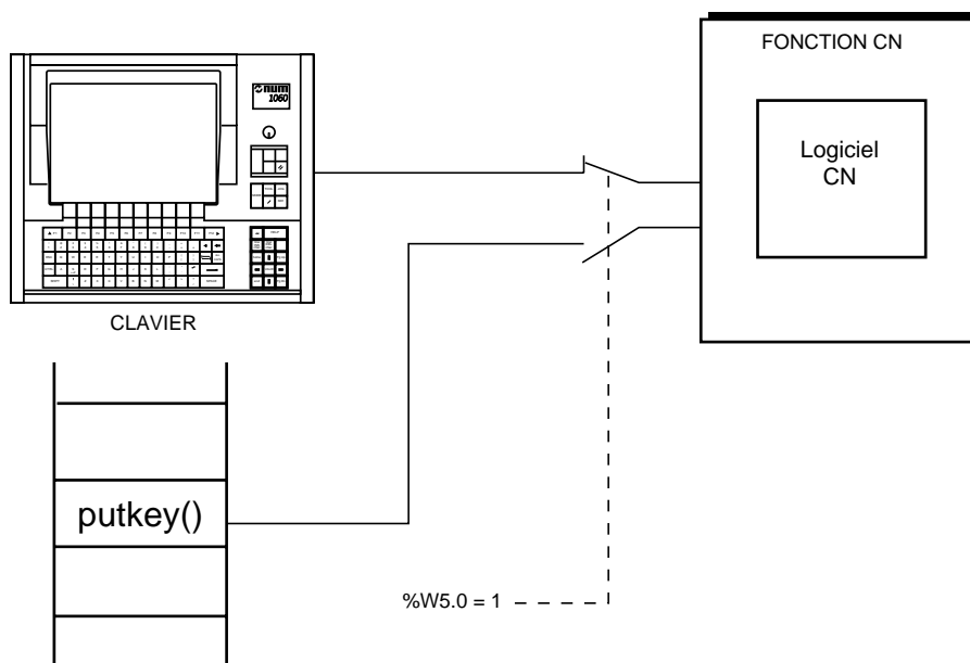
Figure 8.3 - Fonction putkey()
